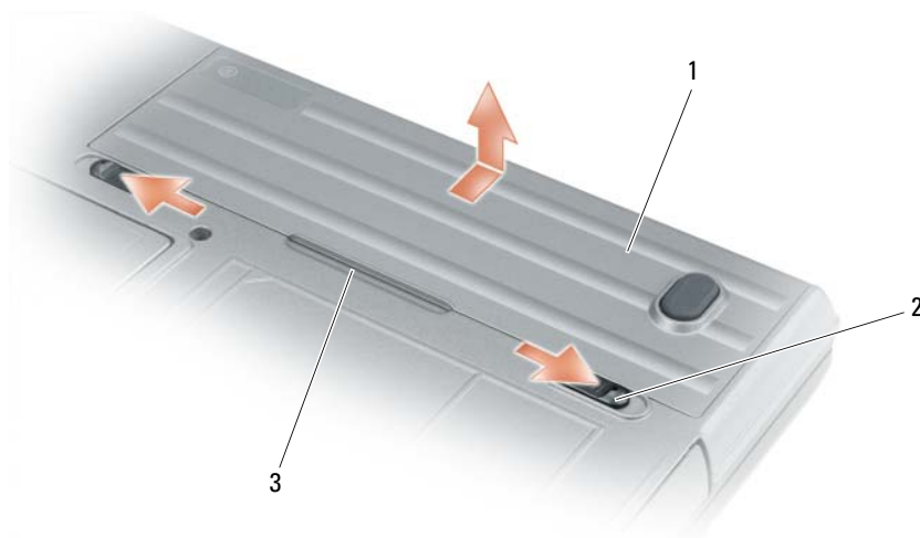
1 电池 2 电池槽释放门锁（2个） 3 电池卡舌
