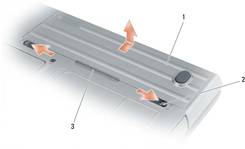
1 전지 2 전지 베이 분리 래치 (2) 3 전지 탭
