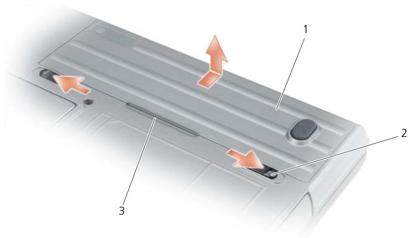
1 バッテリー 2 バッテリーベイリリースラッチ (2) 3 バッテリータブ
